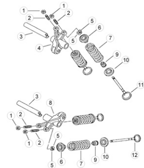
TAV.11A Valvole - Valves - Soupapes - Ventil - Válvulas
