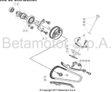
TAV.11B Catena distribuzione - Timing chain - Chaîne de distribution - Steuerkette - Cadena de distribución
