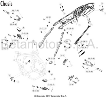
TAV.32 Accessori telaio - Frame accessories - Accessoires chassis - Rahmenzubehören - Accesorios Chasis
