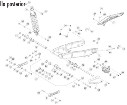
TAV.33 Forcellone posteriore - Rear fork - Fouche arriere - Hinterradschwinge - Horquilla posterior
